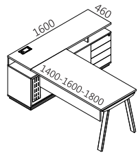
MESA GERENTE C/ ARMÁRIO CREDENZA LD
