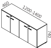
ARMÁRIO 4 PORTAS
